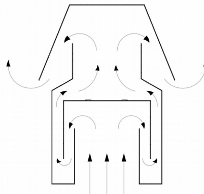
Рисунок 1. Принцип действия искрогасителя.
