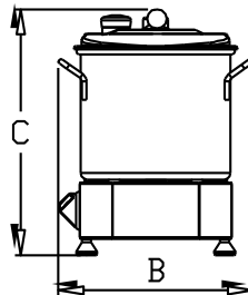
Рис. 1 - Технические параметры измельчителя
