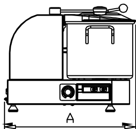
Рис. 1 - Технические параметры измельчителя
