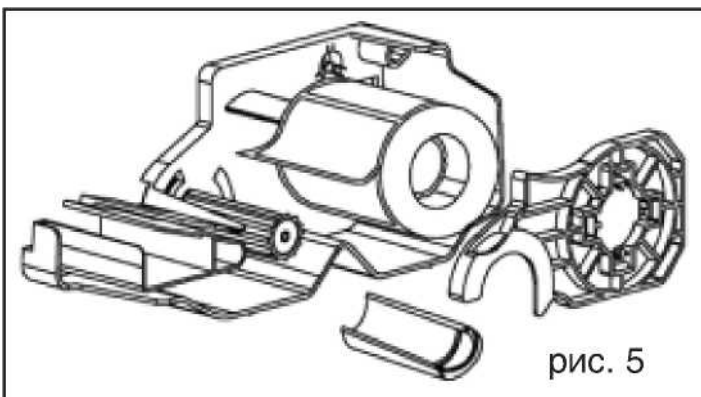
Рисунок 1.15 – Установка рулона
