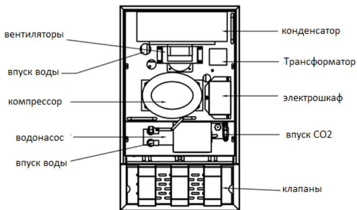
Рис 1 Основные элементы
